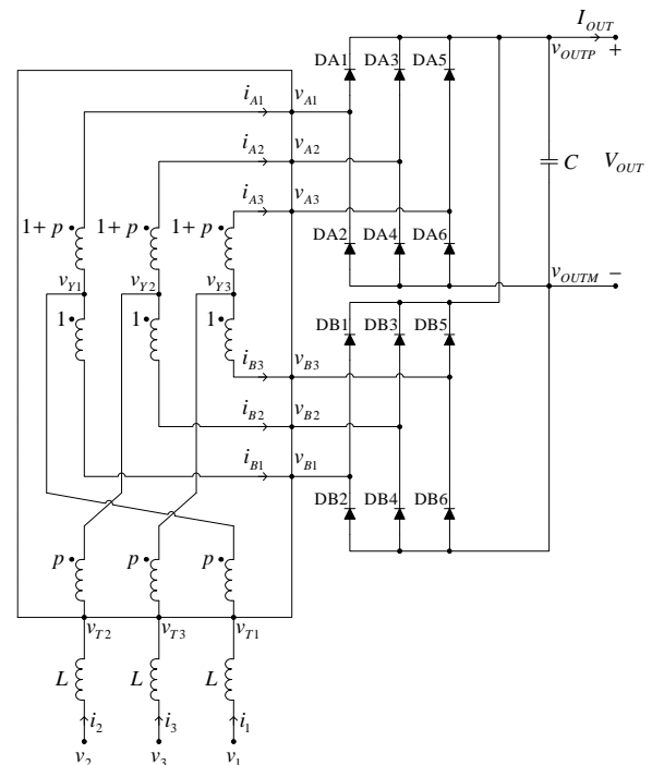
Fig. 1. The rectifier
